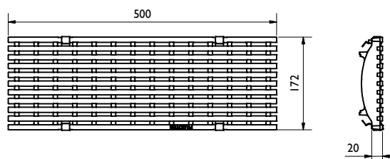
grille décorative en fonte ductile: VILLE, E600 BG code: GJS 17015180; 8,6 kg:
