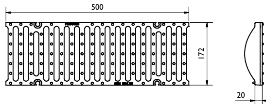
grille à barres longitudinales en fonte ductile: LM22/13, E600 BG code: GJS 17015103; 7,2 kg: 4-fois verrouillable
