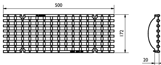
grille à barres longitudinales en fonte ductile: LM22/13, E600 BG code: GJS 17015103; 7,2 kg: 4-fois verrouillable
