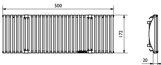
grille décorative en fonte ductile: RIVER, D400 BG code: GJS 17015185; 6,1 kg:
