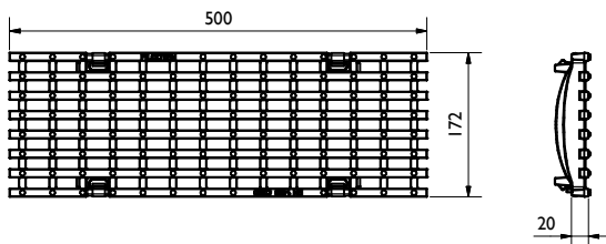
grille décorative en fonte ductile: KIARO, D400 BG code: GJS 17015183; 6 kg:
