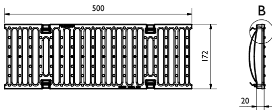
grille à barres longitudinales en fonte ductile: LM25/13, D400 BG code: GJS 17015102; 5,2 kg: 4-fois verrouillable
