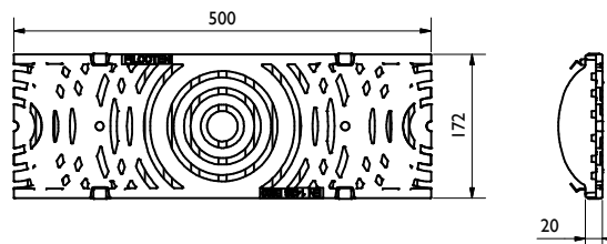
grille à fentes en fonte ductile: LF14/150, D400 BG code: GJS 17015108; 5,5 kg: 4-fois verrouillable
