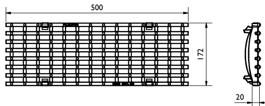
grille décorative en fonte ductile: VIA, D400 BG code: GJS 17015184; 5,6 kg:
