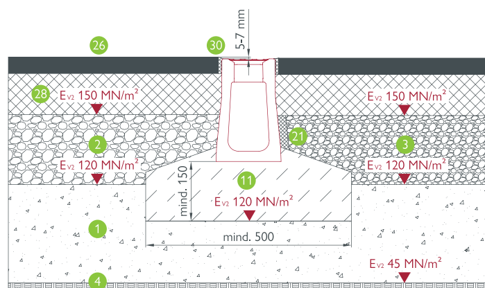
BG-FILCOTEN® one urban, NW 100: Asphalt – Asphalt, Kl. A – C
