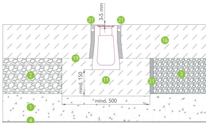
BG-FILCOTEN® one urban, NW 100: Beton – Beton, Kl. A – D urbaner Bereich, mittlere Radlasten
