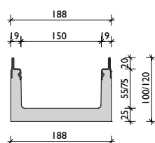
Edelstahlzarge
