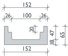
BG-FILCOTEN® city mini 100 inkl. COMBee-Designrost
