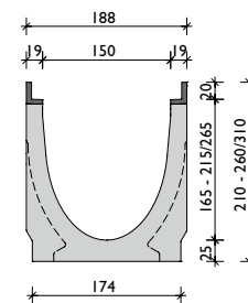
Gusszarge
