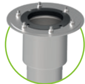
Punktablauf (Edelstahl V2 1.4301) mit senkrechtem Ablauf DN 110
