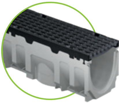
BG-FILCOTEN ® pro G 150 inkl. Gusszarge
