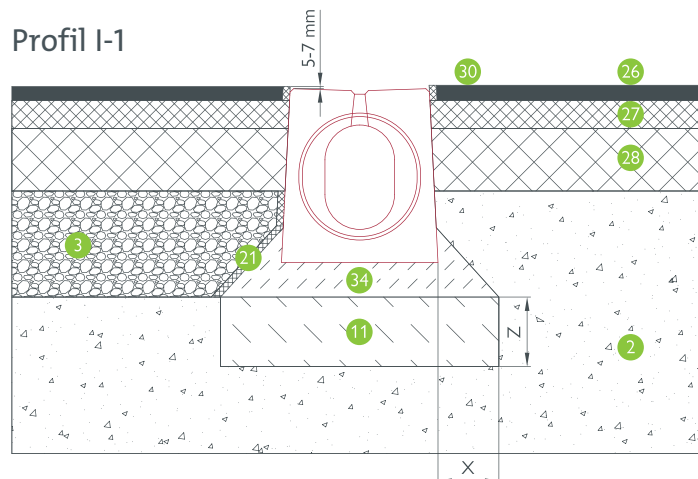
BG-CLASSIC BG-SL, NW 100: Asphalt – Asphalt, Kl. D - F
