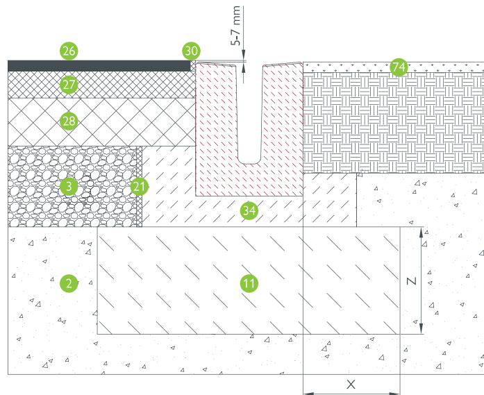
BG-CLASSIC BG-SL, NW 100: Asphalt – Grünfläche, Kl. E- F
