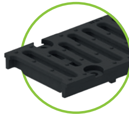
Gussrost SW 16/120 bzw. 16/220, Kl. F – 4-fach verschraubbar, für NW 100 und 200
