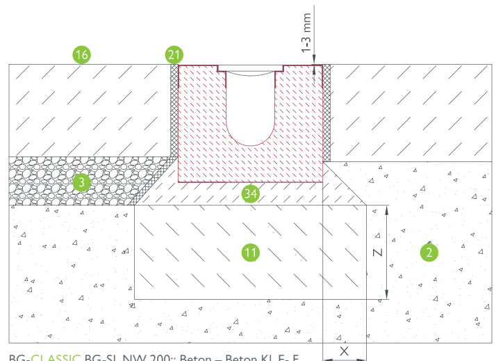
BG-CLASSIC BG-SI, NW 200: Beton – Beton Kl. E- F
