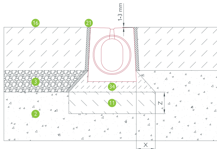
BG-CLASSIC BG-SL, NW 100: Beton – Beton Kl. D - F
