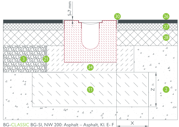
BG-CLASSIC BG-SI, NW 200: Asphalt – Asphalt, Kl. E- F
