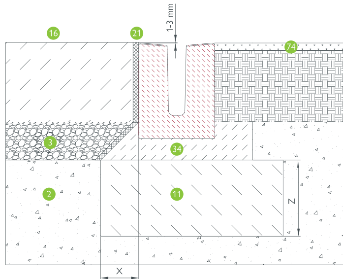
BG-CLASSIC BG-SL, NW 100: Beton – Grünfläche, Kl. E- F
