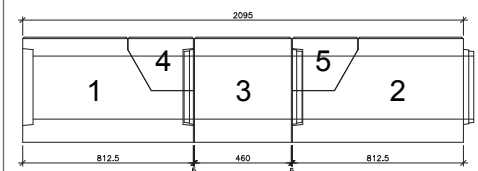
Skizze Austauschelement
