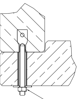
Gewindestange, Unterlagscheibe und Sechskant-Mütter M24 (SW 36)
